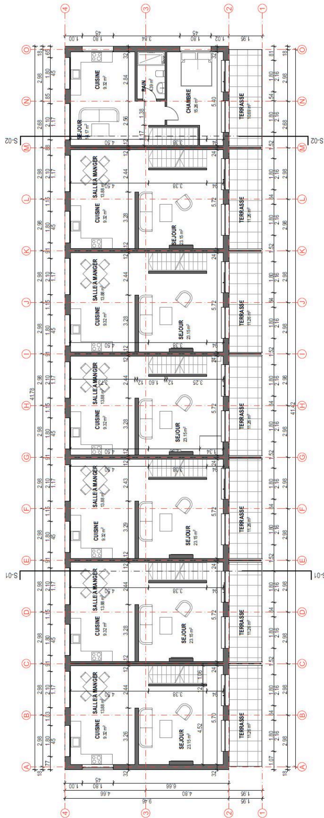
ÉTAGE 1
